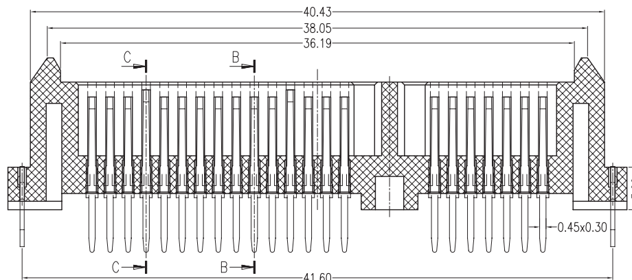
SECT A-A
