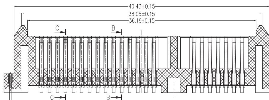
SECT A-A
